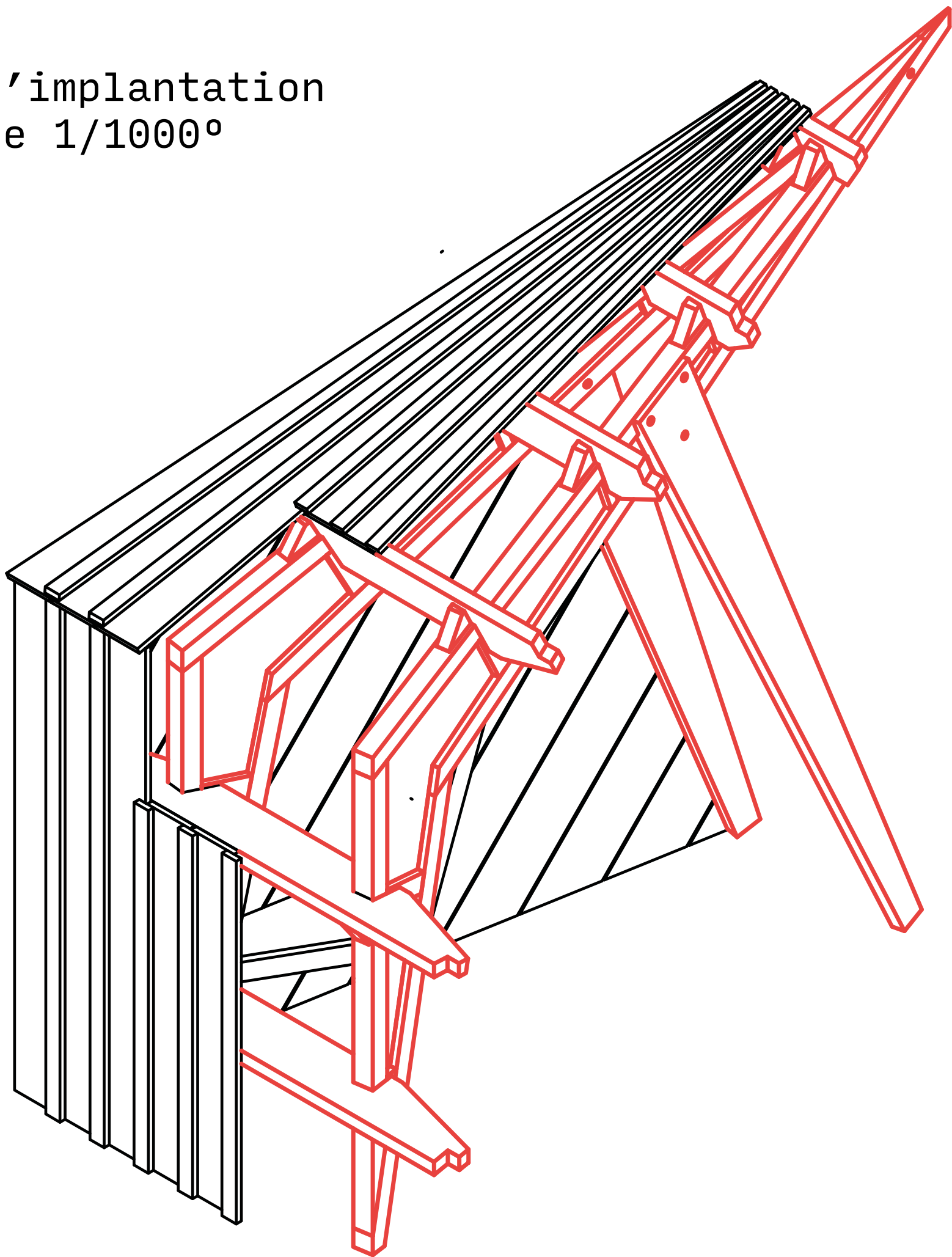
Écorché isométrique de la structure
