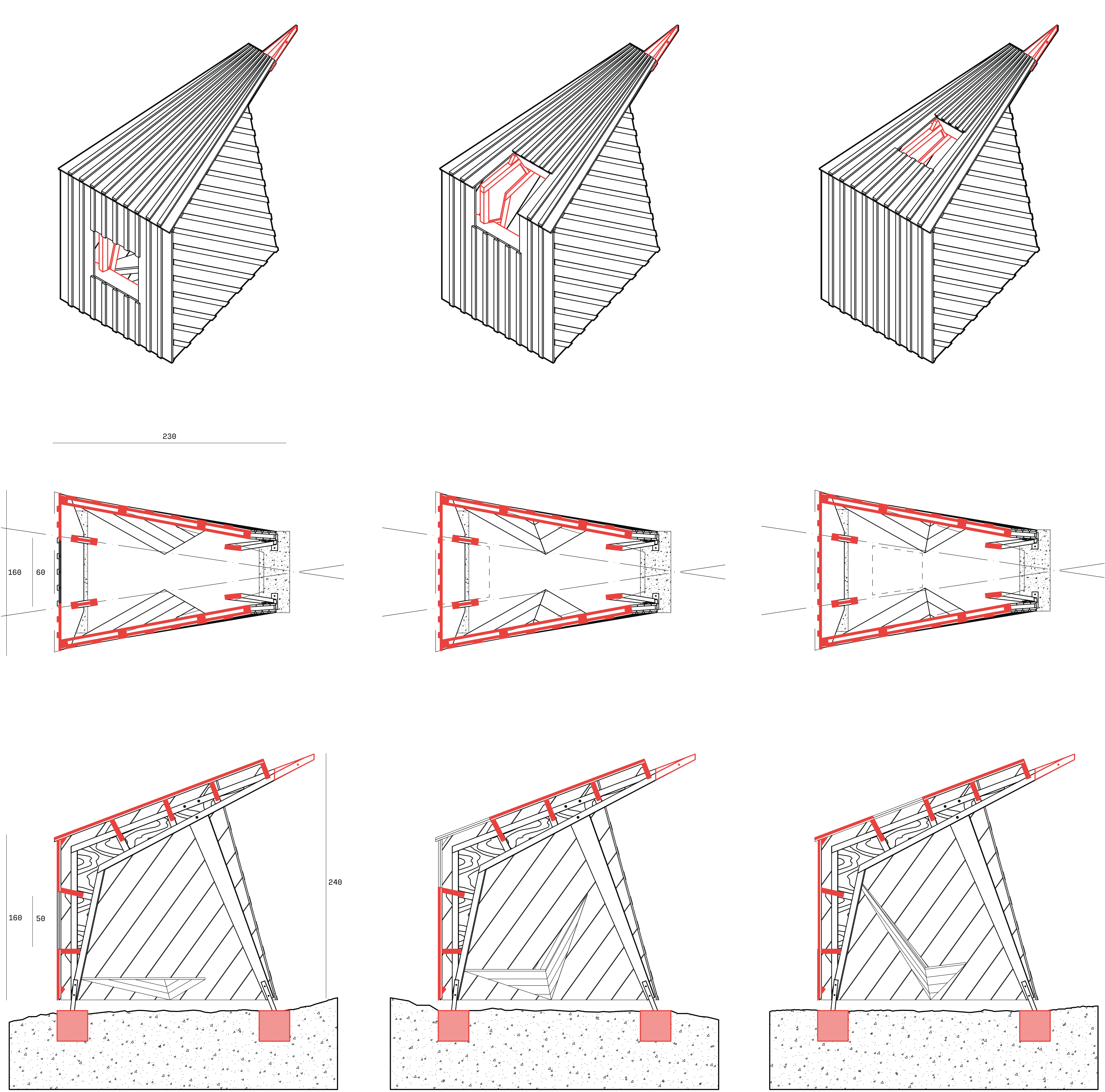
Plans, coupes et axonométries des confessionnaux - échelle 1/20°
