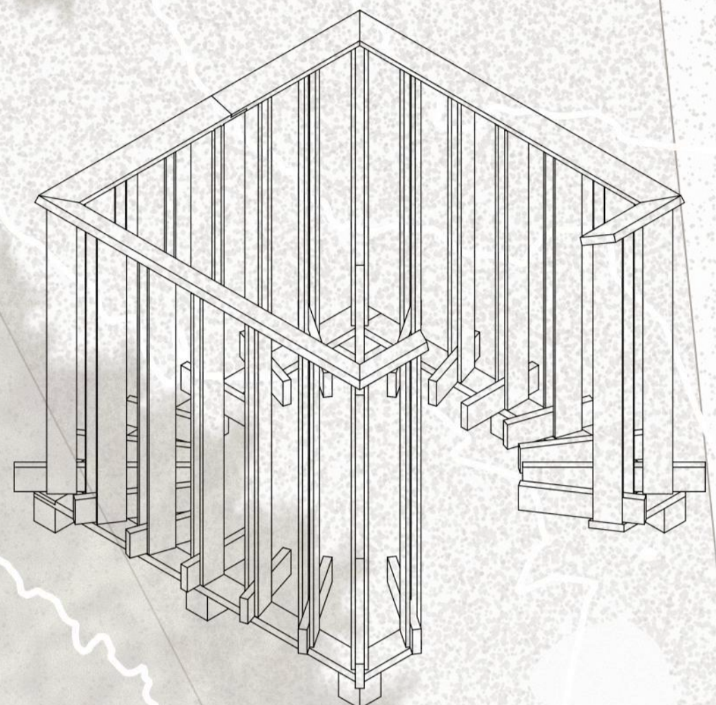
Fixation de la lisse haute
