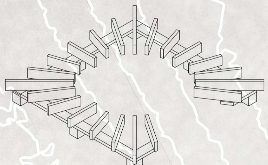
Fixation pannes sur la lisse basse
